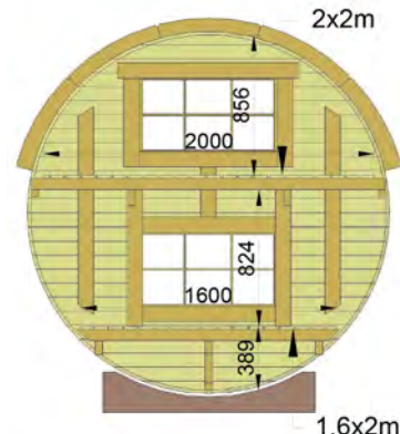
- TONNEAU Ø 2.2 x 4.4 m - Solution A et B
