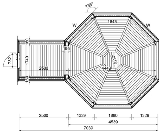
Avec l'extension de 4.30 m 2 : Longueur 7.04 m
