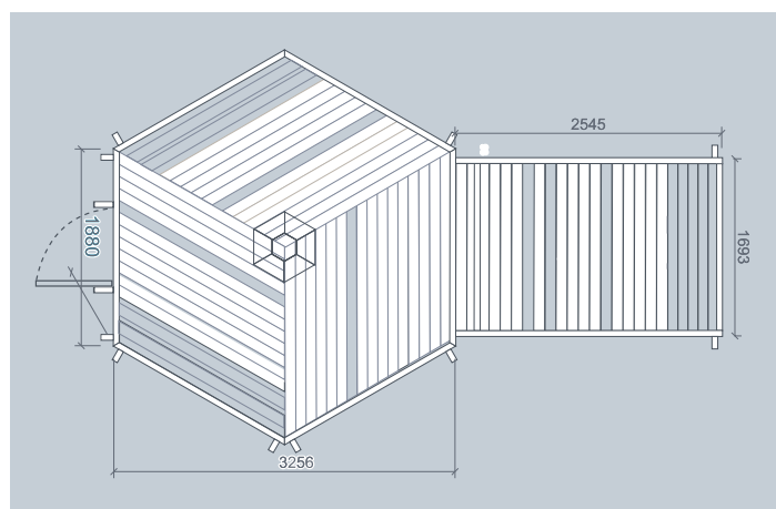
Avec l'extension de 4.30 m 2 : Longueur 5.80 m
